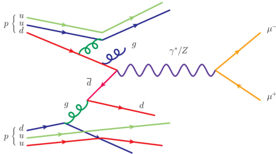
Slika 1.2: Feynmanov dijagram Drell-Yan procesa. Izvor: [4]
