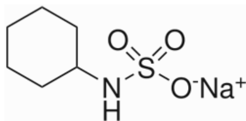
Slika 5. Kemijska struktura ciklamata ( C_6H_{12}NNaO_3S )
