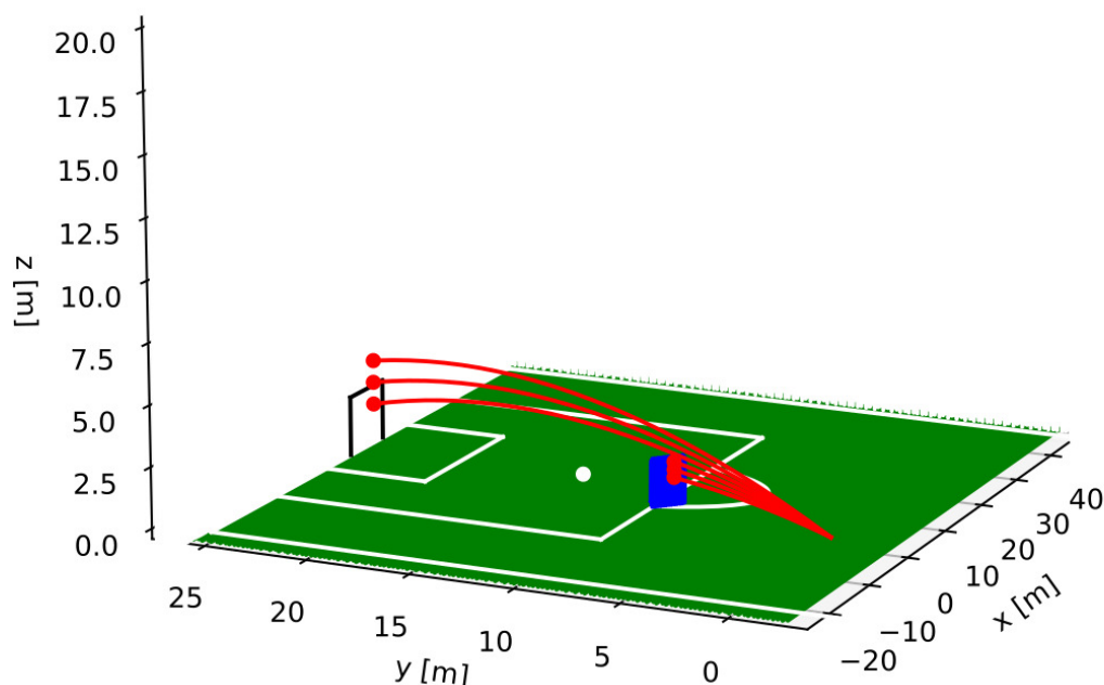
Slika 9: Učinkovitost obrambenog zida ( H = 2 \text{ m} , L = 3 \text{ m} ) testirana je ispaljivanjem lopte s položaja koji odgovara \mathbf{s} = (10 \text{ m}, 25 \text{ m}) . Ispaljivane su lopte pod različitim kutevima \vartheta , svaka s topspinom koji odgovara \Delta\vartheta = 2^\circ . Za sve putanje vrijedi \varphi = 60^\circ , \Delta\varphi = 0^\circ
